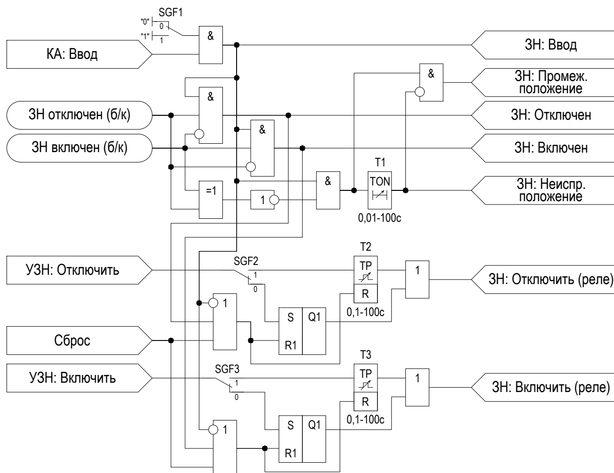
Рисунок 2.66 – Функциональная схема «3Н»
